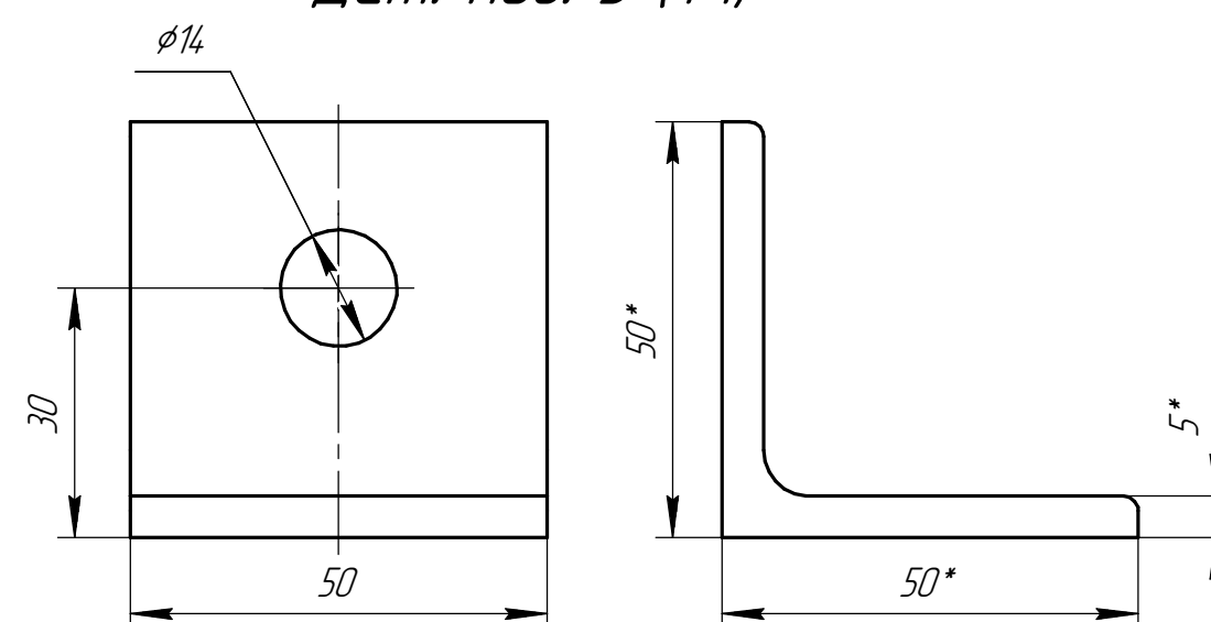
Дет. поз. 5 (1:1)
