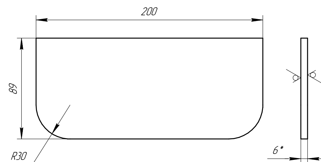
Дет. поз. 2 (1:2)
